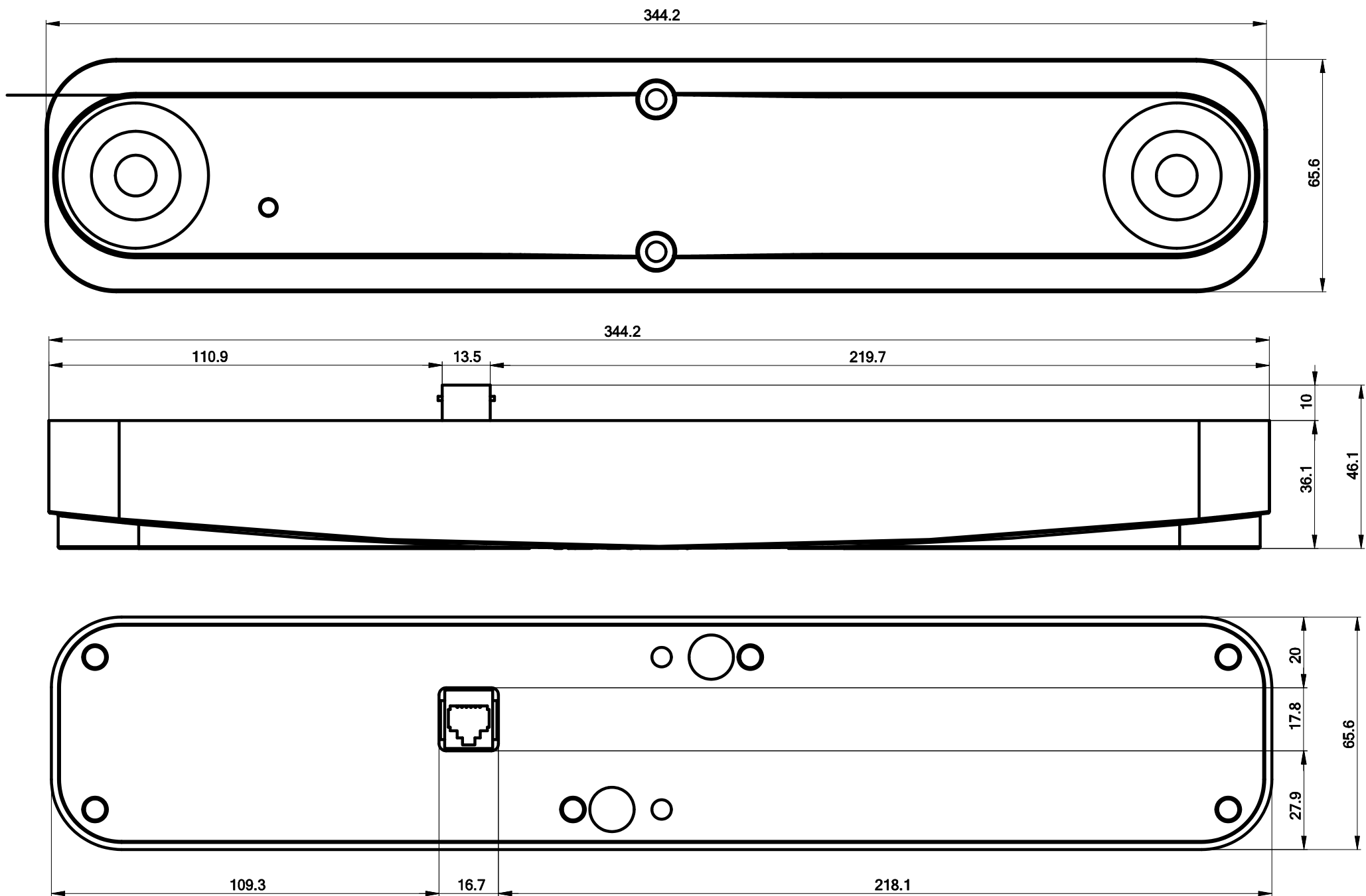
Abmessungen Xovis PC3 Zählsensoren
