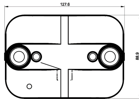
Abmessungen Xovis PC2
